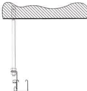
Rys. 1 Koryto siatkowe GRM 55 50 zamontowane na prętach przy użyciu uchwyty SHU M12; podpory co 1,5m, obciążenie maks. 3kg/m
