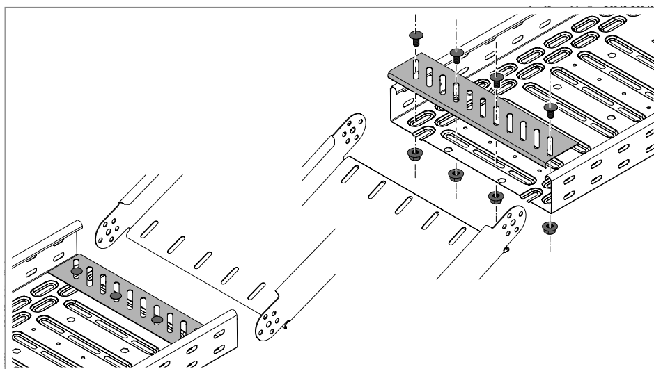
Rys. 70: Montaż dennej blachy końcowej
