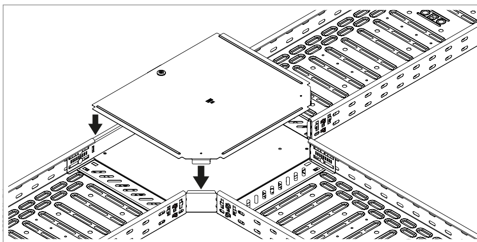
Rys. 90: Nakładanie pokryw kształtek
