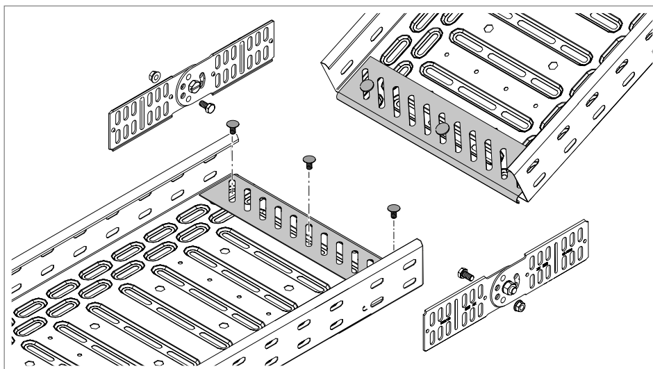
Rys. 39: Przykręcanie dennych blach końcowych
