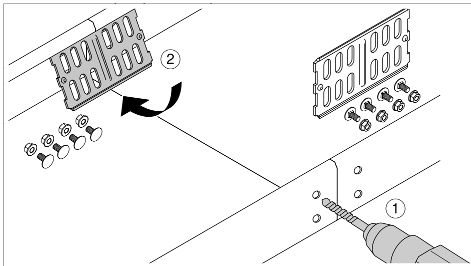
Rys. 25: Zakładanie łącznika wzdłużnego RLVK
