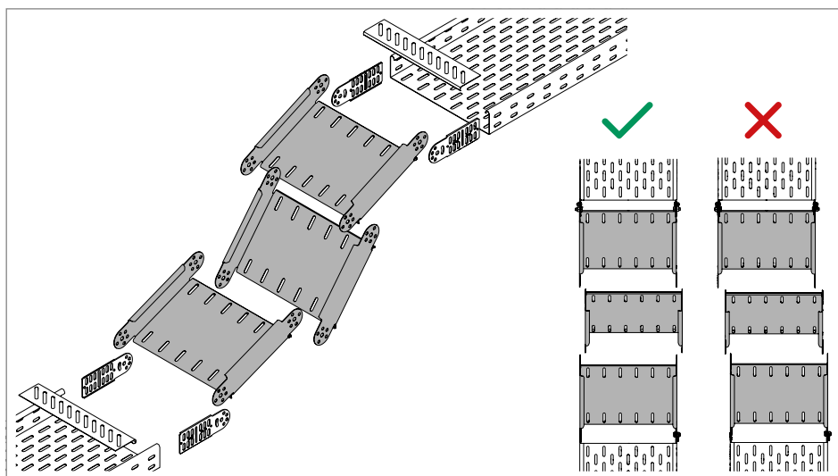
Rys. 69: Element łuku przegubowego z połówką łącznika przegubowego i denną blachą końcową
