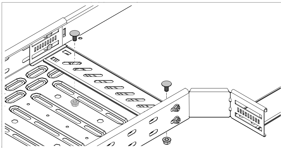
Rys. 54: Przykręcanie listwy stykowej
