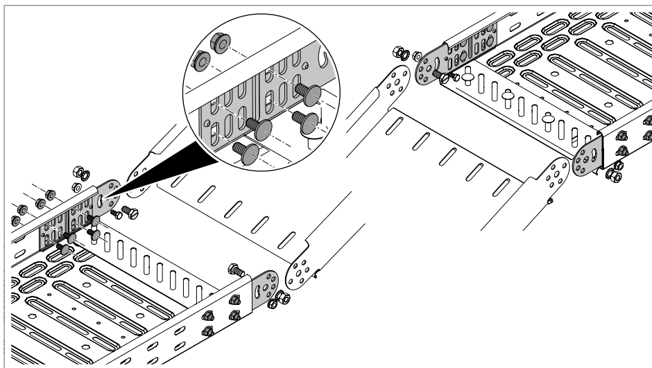
Rys. 71: Montaż łączników przegubowych na korytkach kablowych
