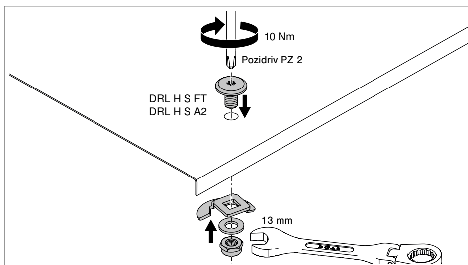
Rys. 87: Przykręcanie rygla obrotowego
