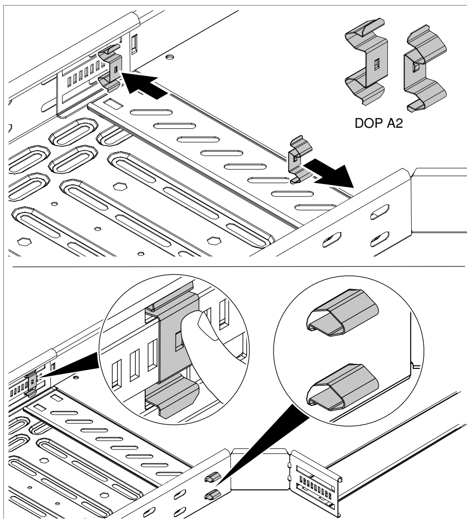
Rys. 51: Mocowanie kształtki zaciskiem podwójnym
