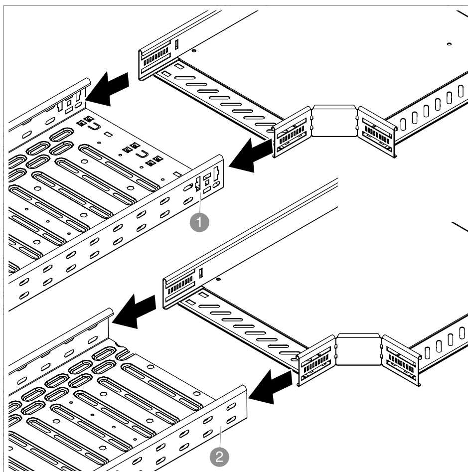
Rys. 45: Wsuwanie kształtki
