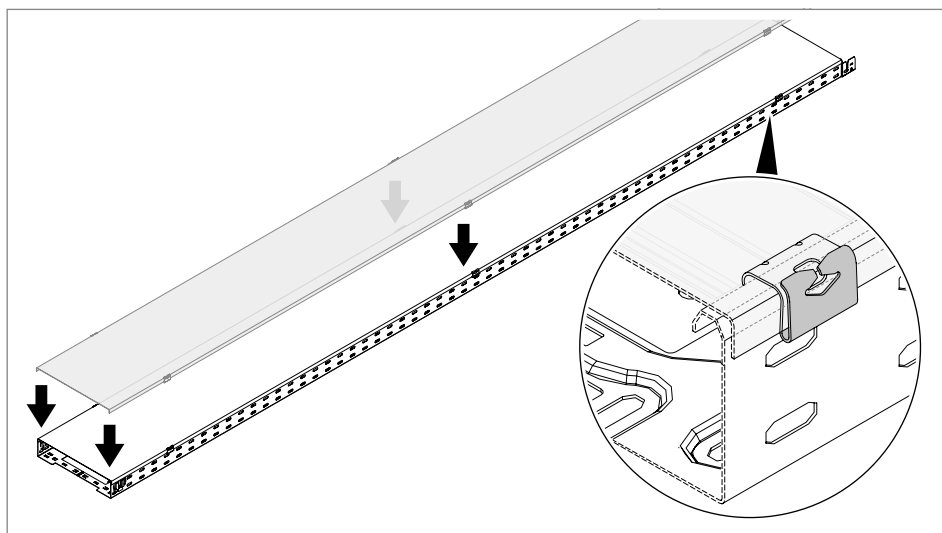
Rys. 85: Zatraskiwanie pokrywy
