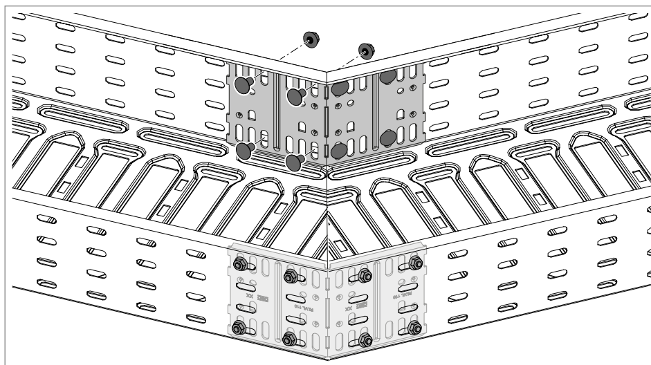
Rys. 32: Przykręcanie łącznika wzdłużno-kąowego RLVL
