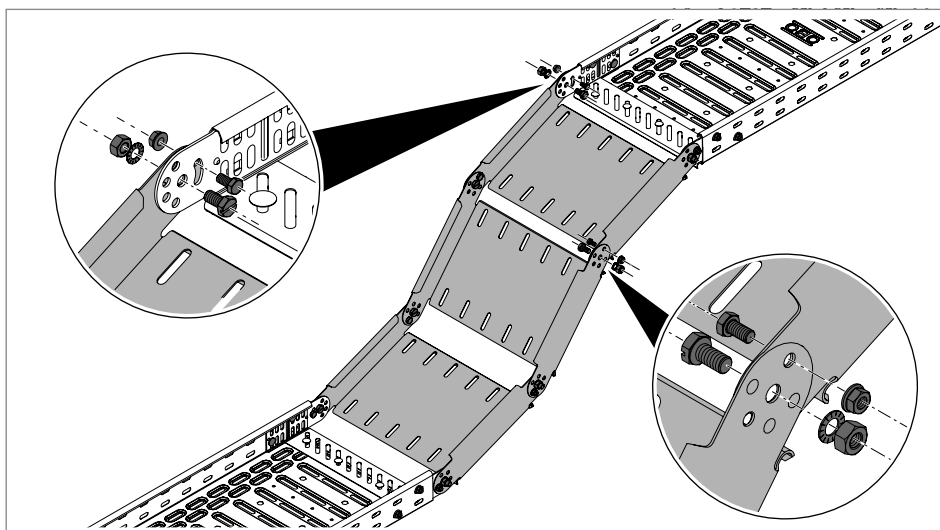
Rys. 72: Montaż elementów łuku przegubowego
