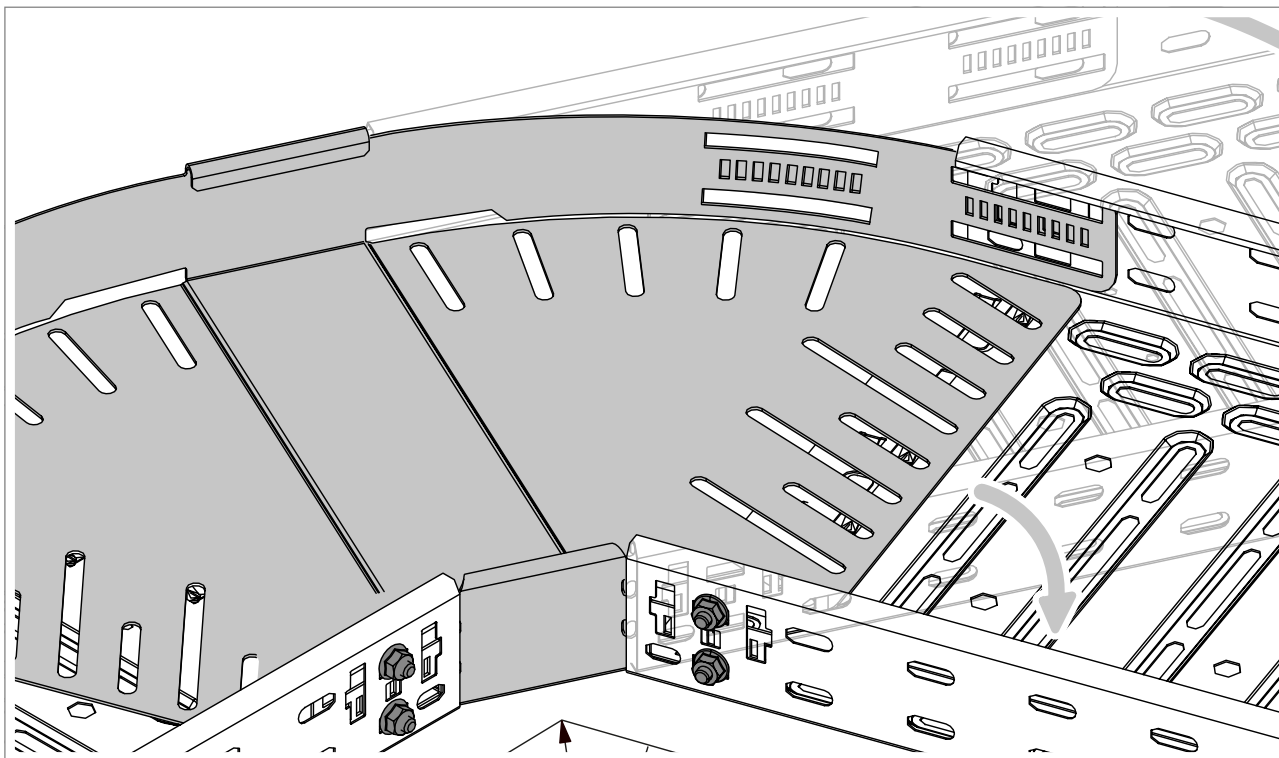
Abb. 65: Zaginanie korytek wokół łącznika wewnętrznego
