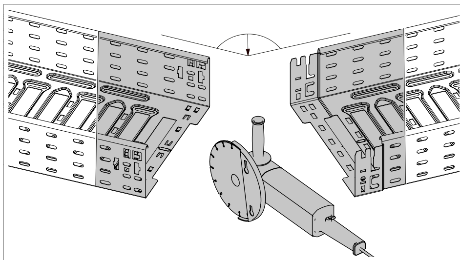
Rys. 30: Przycinanie korytka kablowego do ustawienia kąтового
