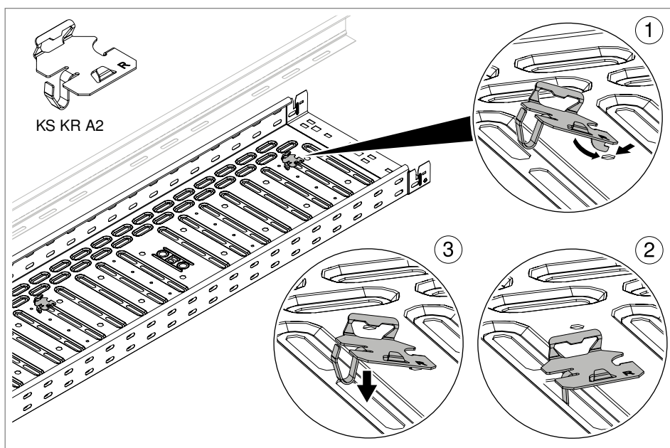
Rys. 79: Zakładanie zacisku przegrody
