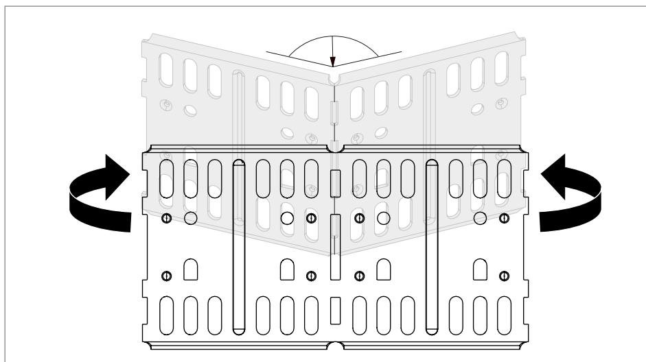
Rys. 31: Zaginanie łącznika wzdłużno-kąowego RLVL
