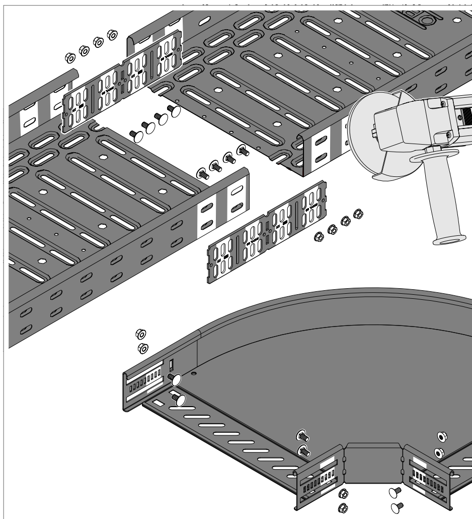
Rys. 18: Usuwanie powłoki proszkowej
