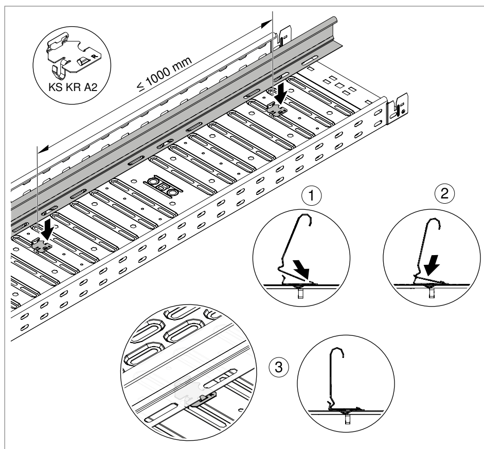
Rys. 80: Mocowanie przegrody w zacisku
