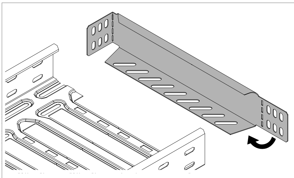
Rys. 76: Zaginanie zacisku
