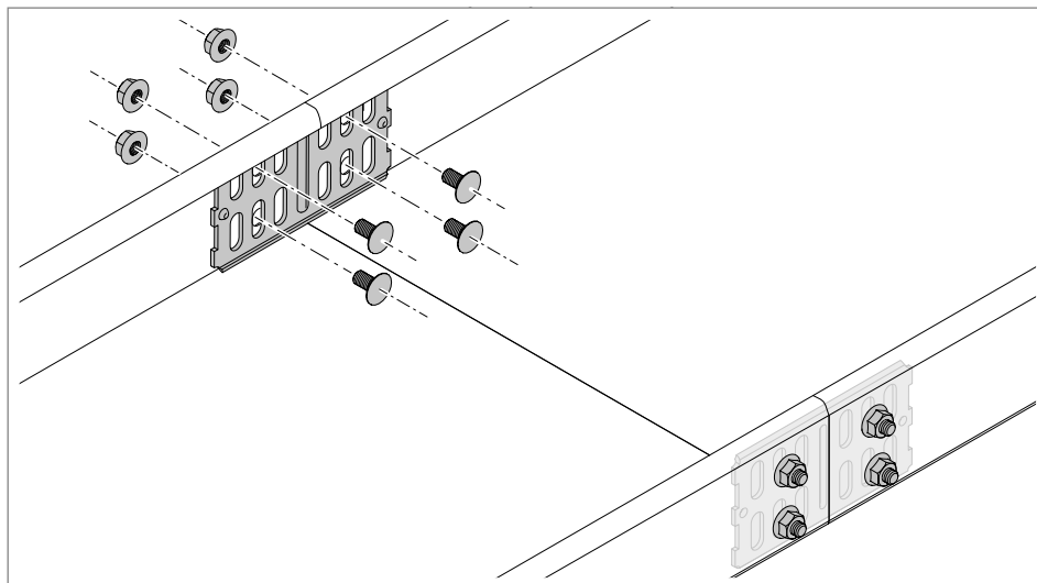
Rys. 26: Dokręcić łącznik wzdłużny RLVK
