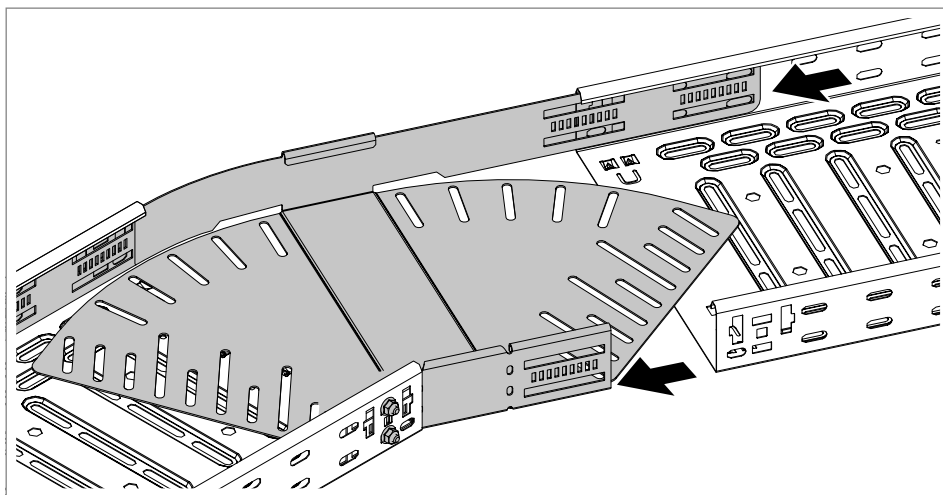
Rys. 63: Nasuwanie drugiego korytka na łuk
