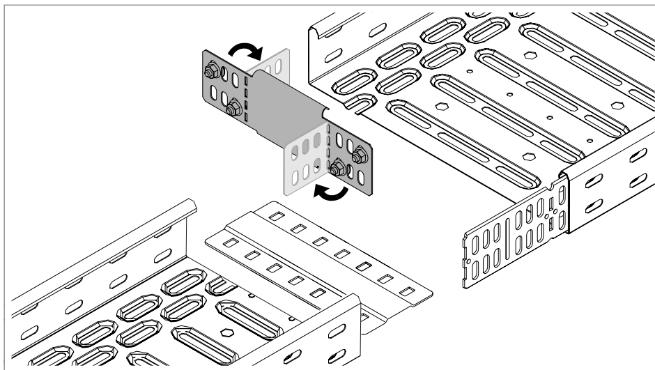
Rys. 73: Zaginanie kątownika redukcyjnego
