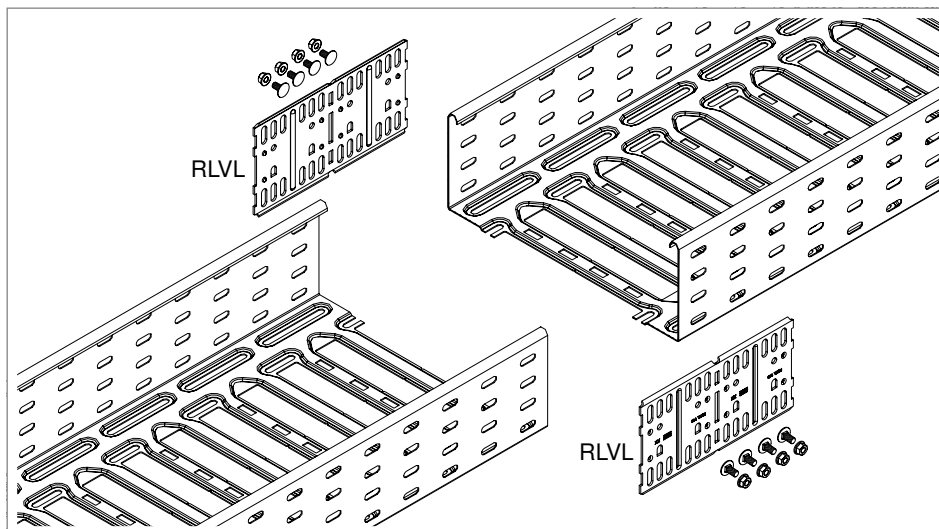
Rys. 27: Łącznik wzdłużny RLVL
