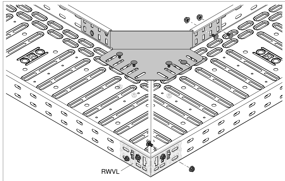
Rys. 37: Montaż łącznika narożnego REV
