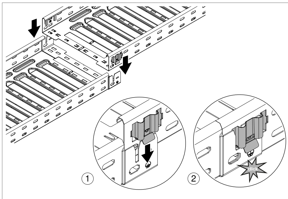
Rys. 19: Połączenie zatraskowe Magic z elementem sprężynowym
