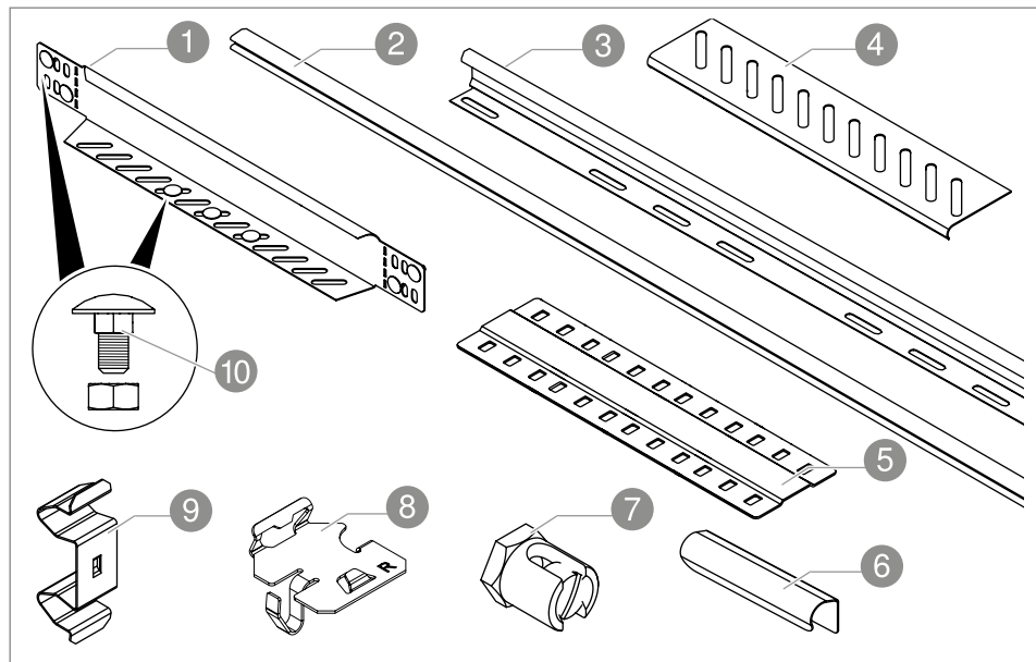
Rys. 15: Osprzęt
