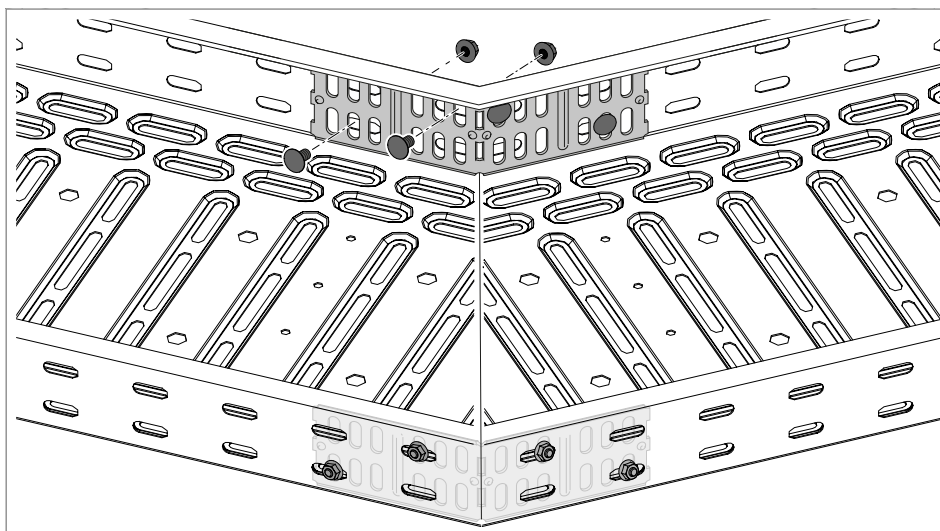
Rys. 35: Przykręcanie łącznika kąтового RWVL
