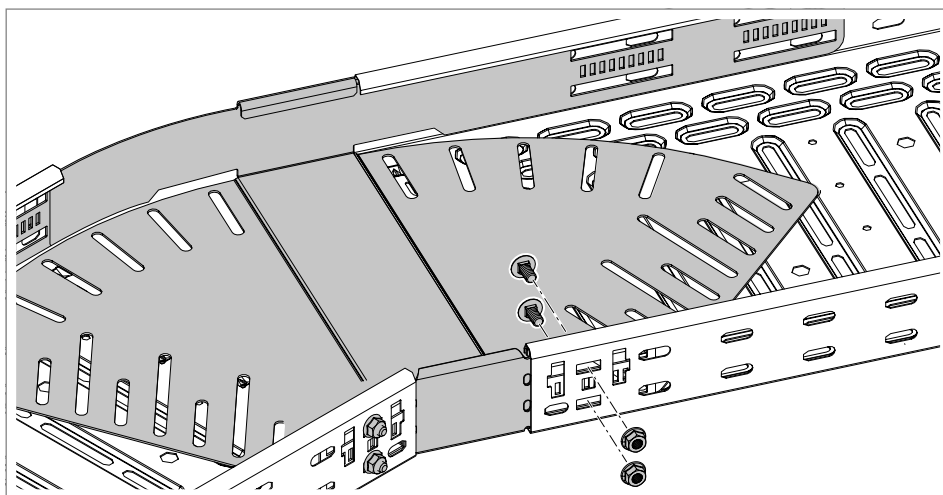
Rys. 64: Mocowanie drugiego korytka do łuku
