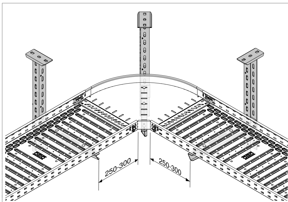
Rys. 44: Przykład: podparcie łuku 90° o szerokości od 400 mm
