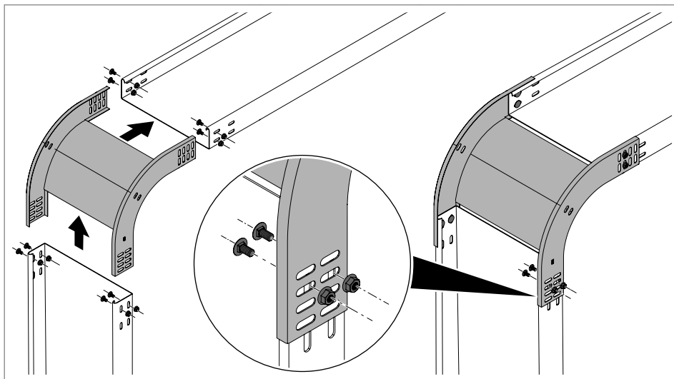
Rys. 67: Montaż opadających łuków pionowych
