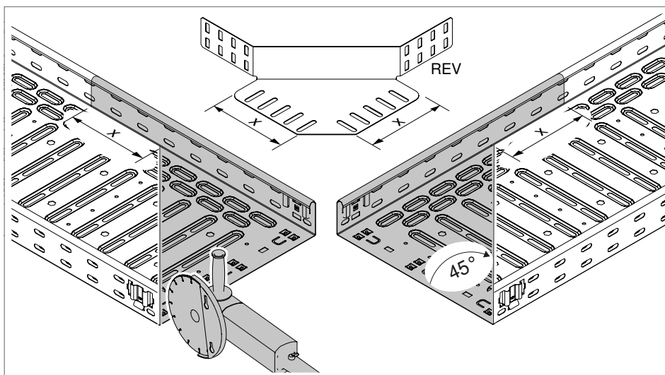
Rys. 36: Przycinanie korytka kablowego do łącznika narożnego REV
