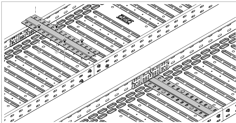
Rys. 16: Montaż listwy stykowej
