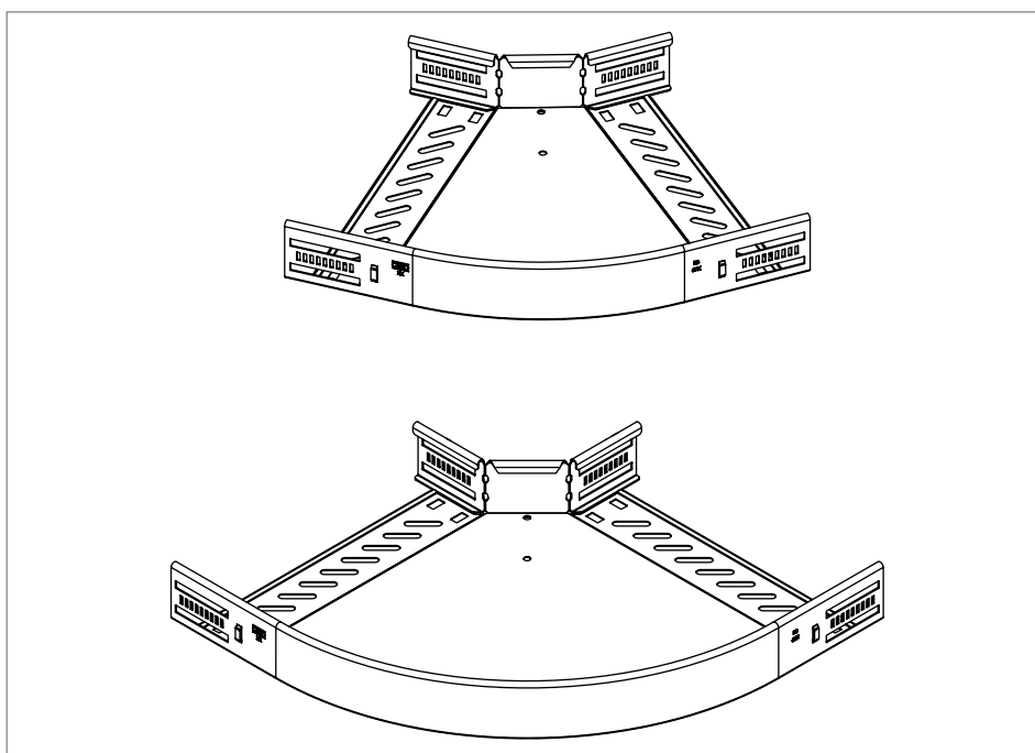
Rys. 3: Łuki 45° i 90°
