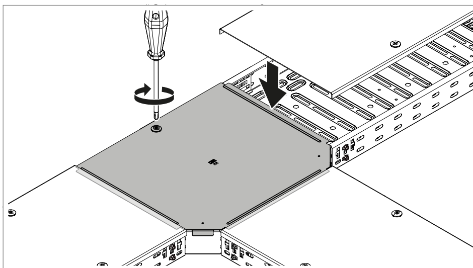
Rys. 91: Zabezpieczanie pokryw kształtek pokrywami odcinków
