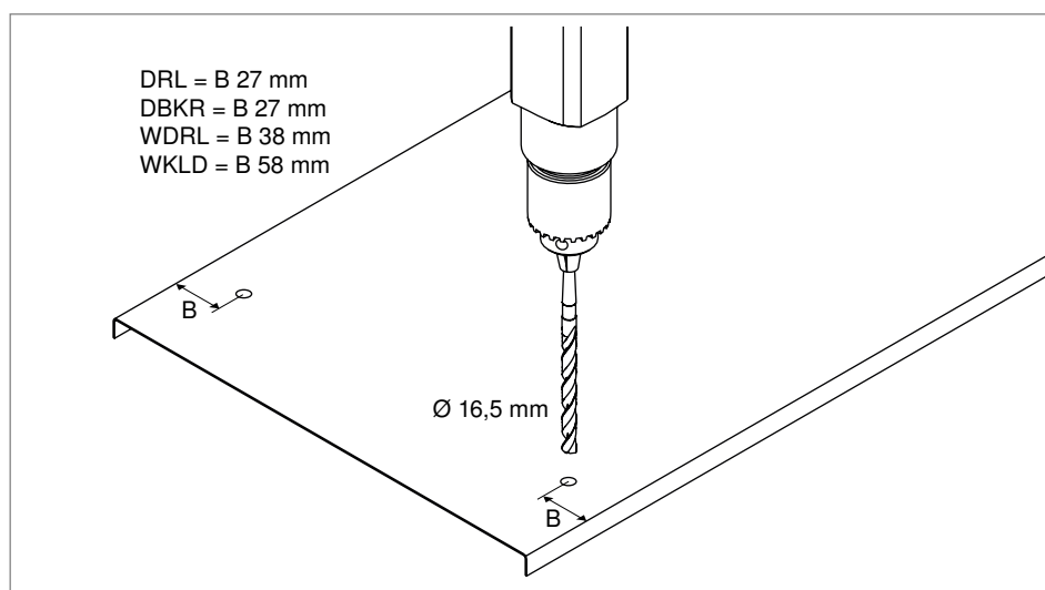
Rys. 86: Wstępne nawiercanie pokryw
