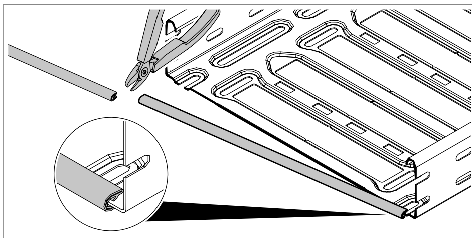
Rys. 17: Montaż taśmy ochronnej krawędzi
