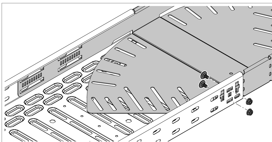
Rys. 61: Mocowanie łuku regulowanego
