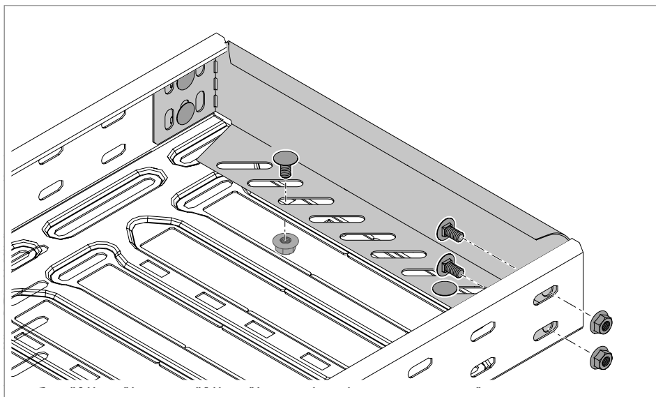
Rys. 77: Montaż zaślepki końcowej
