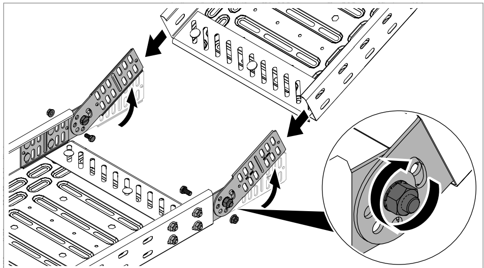
Rys. 41: Dokręcanie śruby przegubowej
