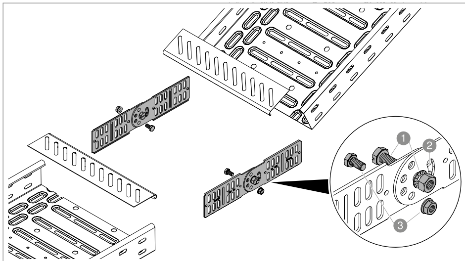
Rys. 38: Łącznik przegubowy RGV i denne blachy końcowe
