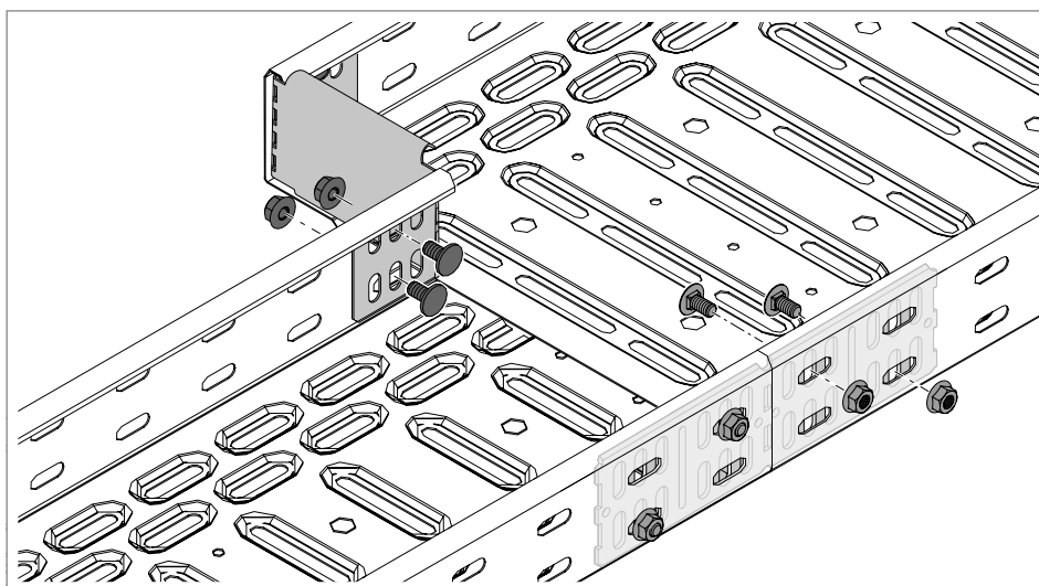
Rys. 74: Montaż łącznika wzdłużno-kątownego i kątownika redukcyjnego
