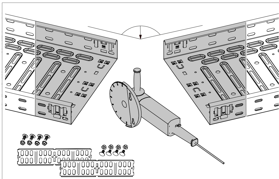
Rys. 33: Przycinanie korytka kablowego do ustawienia kąтового
