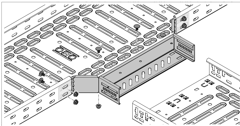
Rys. 56: Przykręcanie trójnika dostawnego do przelotowego korytka kablowego
