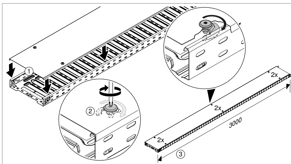
Rys. 89: Montaż pokrywy z ryglem obrotowym Helix
