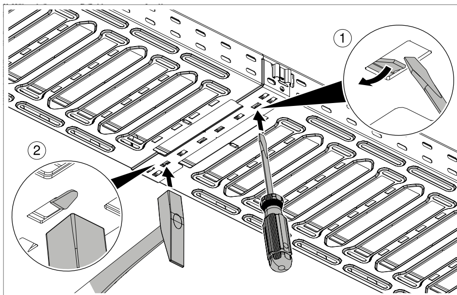
Rys. 20: Zabezpieczanie połączeń korytek
