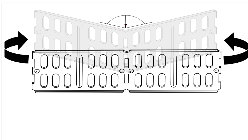
Rys. 34: Zaginanie łącznika kątovej RWVL
