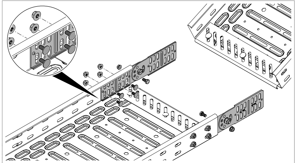
Rys. 40: Przykręcanie łącznika przegubowego RGV do korytka kablowego
