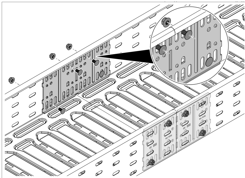
Rys. 29: Dokręcanie łącznika wzdłużnego RLVL
