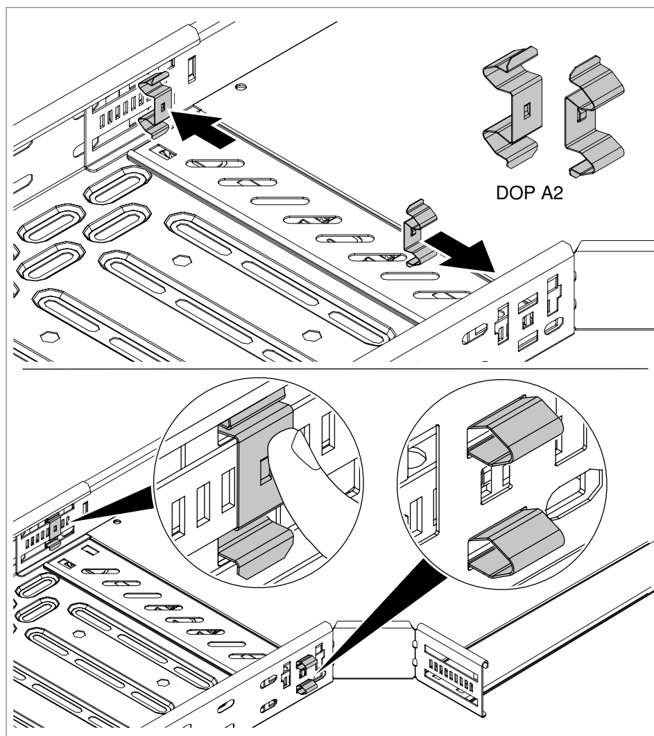
Rys. 46: Mocowanie kształtki zaciskiem podwójnym
