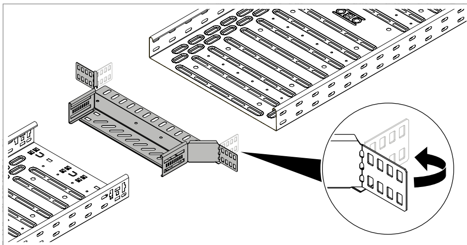
Rys. 58: Zaginanie nakładek łączących
