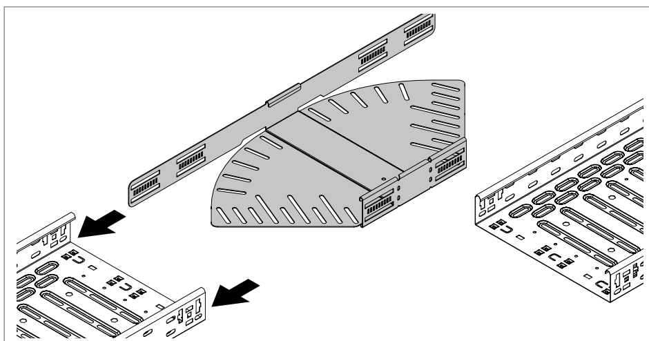
Rys. 60: Wsuwanie łuku regulowanego
