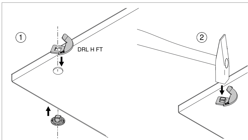
Rys. 88: Nitowanie rygla obrotowego
