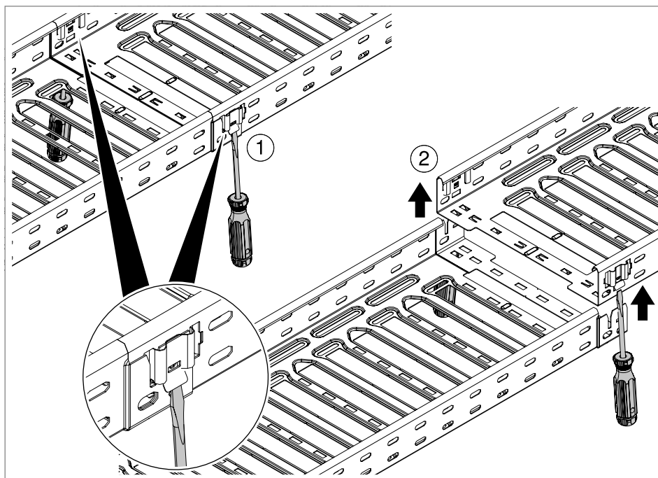
Rys. 92: Rozłączanie połączenia zatraskowego Magic
