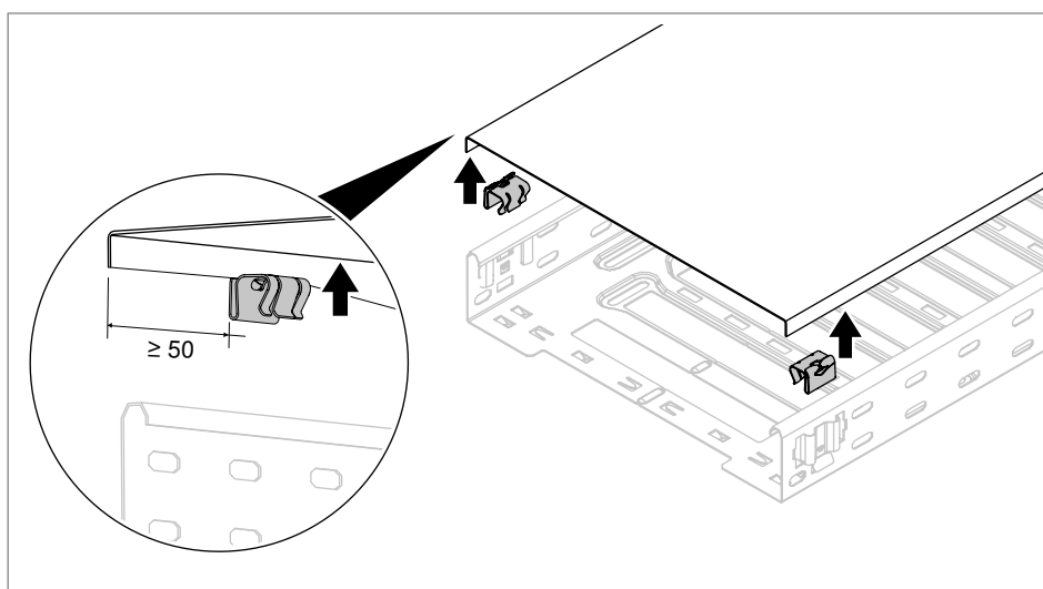
Rys. 83: Zaciskanie klamer na pokrywie
