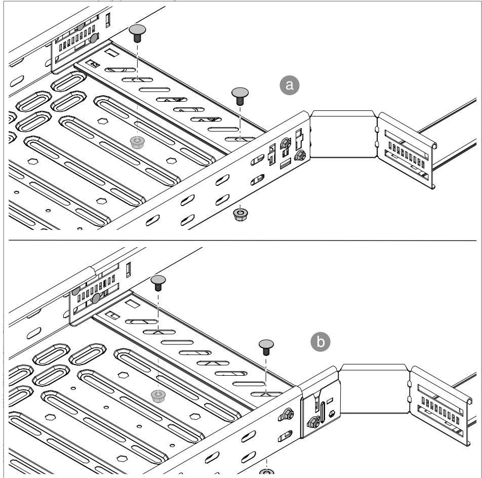
Rys. 50: Przykręcanie listwy stykowej (koniec korytka kablowego a i b )
