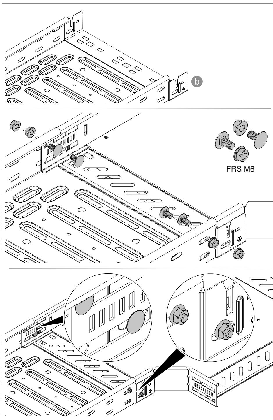
Rys. 49: Mocowanie kształtki śrubami (koniec korytka kablowego (b))
