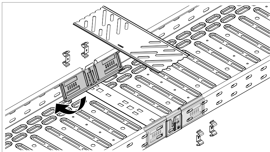
Rys. 22: Zakładanie łącznika wzdłużnego KTSM
