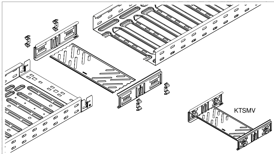
Rys. 21: Łącznik wzdłużny KTSM
