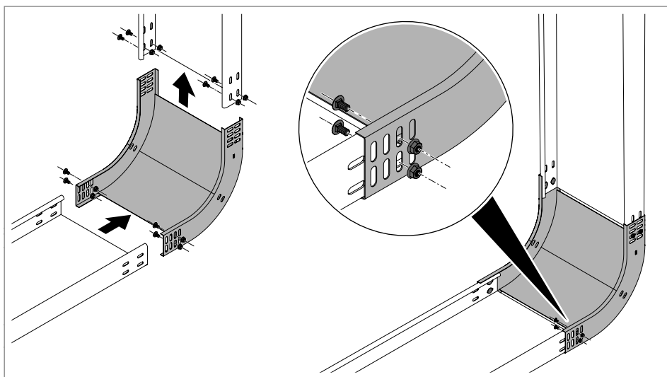
Rys. 68: Montaż wznoszących się łuków pionowych
