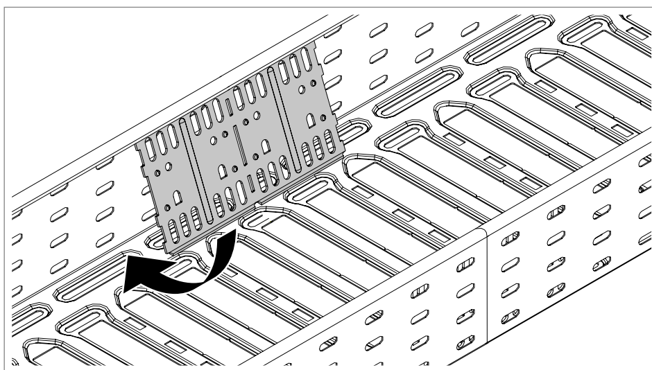
Rys. 28: Stosowanie łącznika wzdłużnego RLVL
