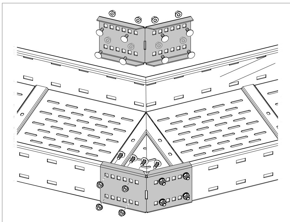
Rys. 18: Przykręcanie łącznika kąтового WRWVK do narożnika wewnętrznego i zewnętrznego
