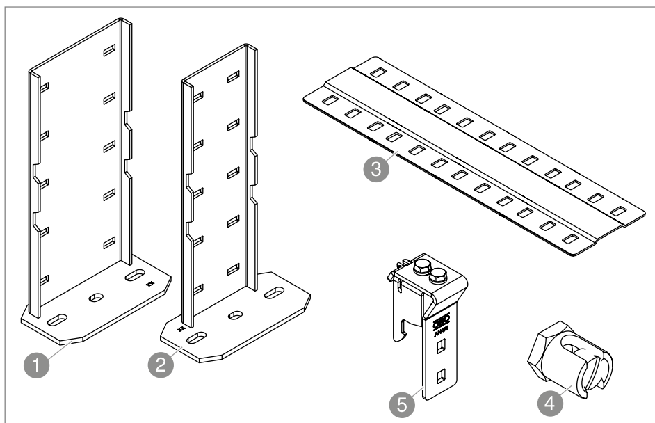
Rys. 9: Osprzęt
