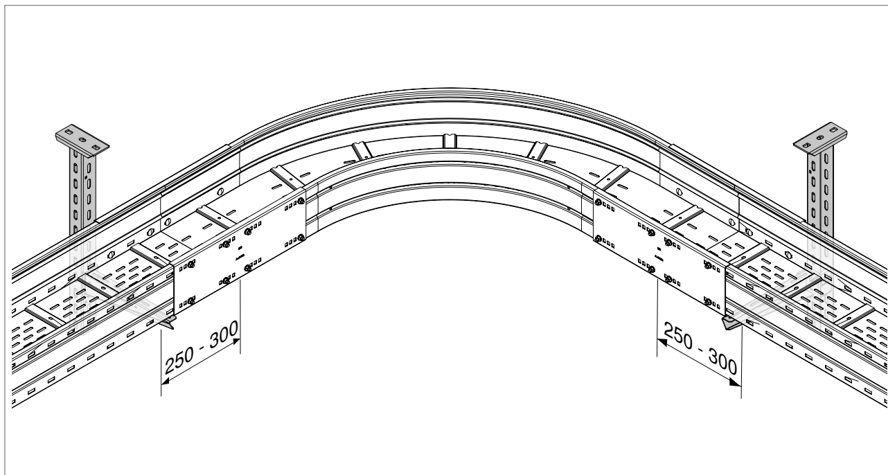
Rys. 30: Przykład: podparcie łuku 90° o szerokości 300 mm
