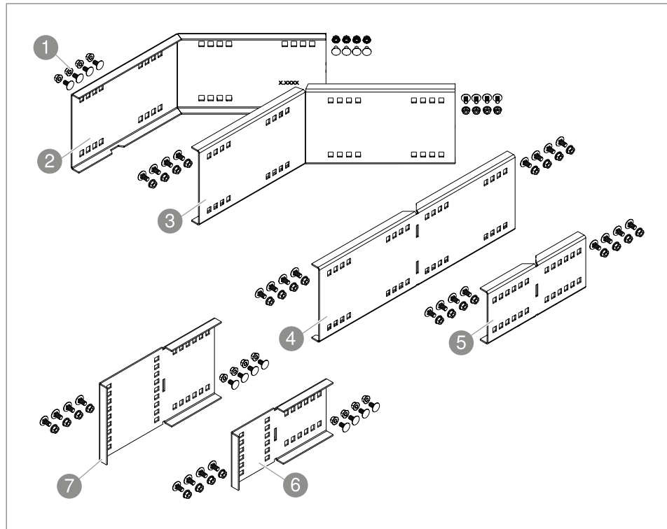
Rys. 3: Łącznik kątowy
