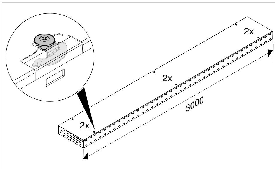
Rys. 46: Zamontowana pokrywa ze wstępnie zamontowanymi ryglami obrotowymi
