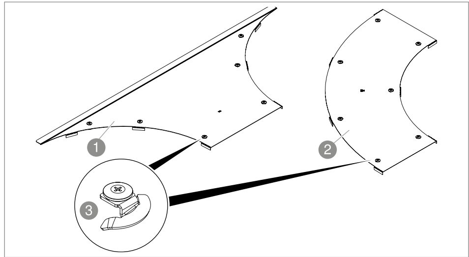
Rys. 8: Pokrywy kształtek
