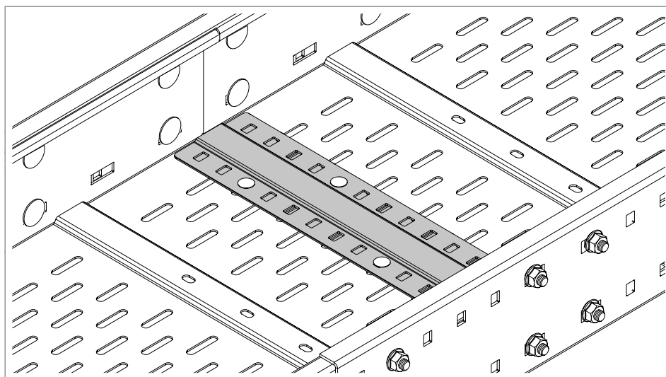
Rys. 13: Zamontowane listwy stykowe
