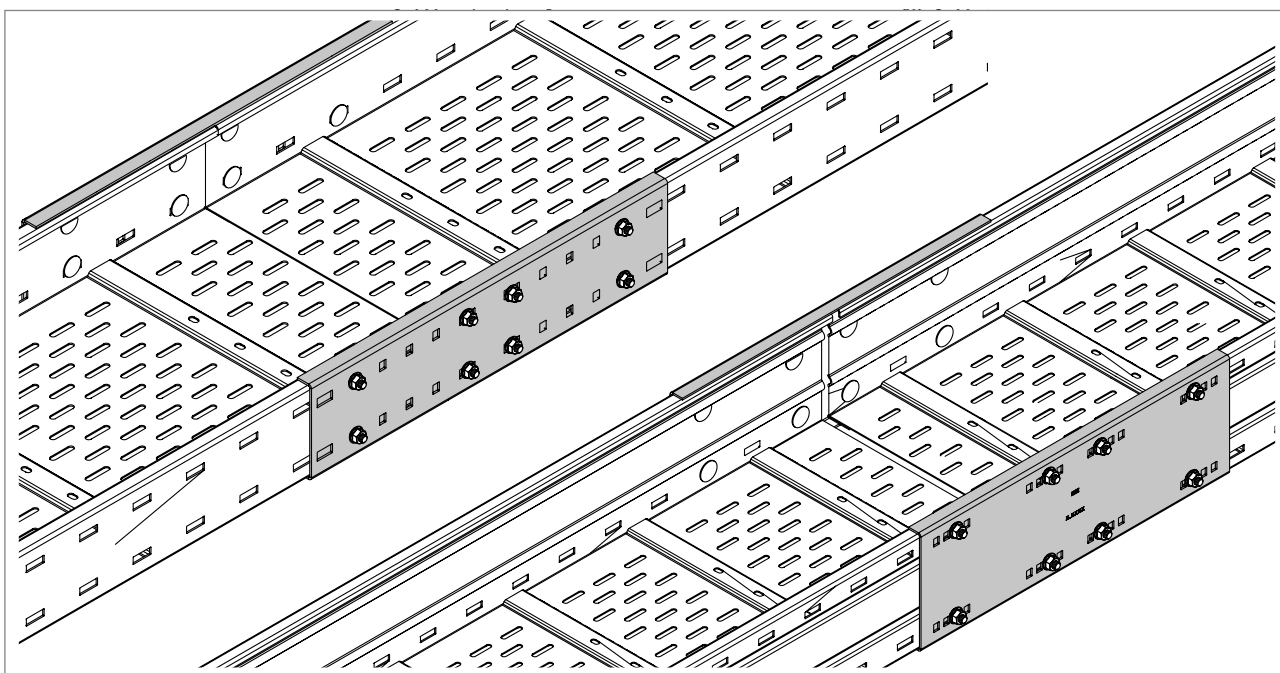
Rys. 11: Dokręcanie łącznika wzdłużnego WRVL
