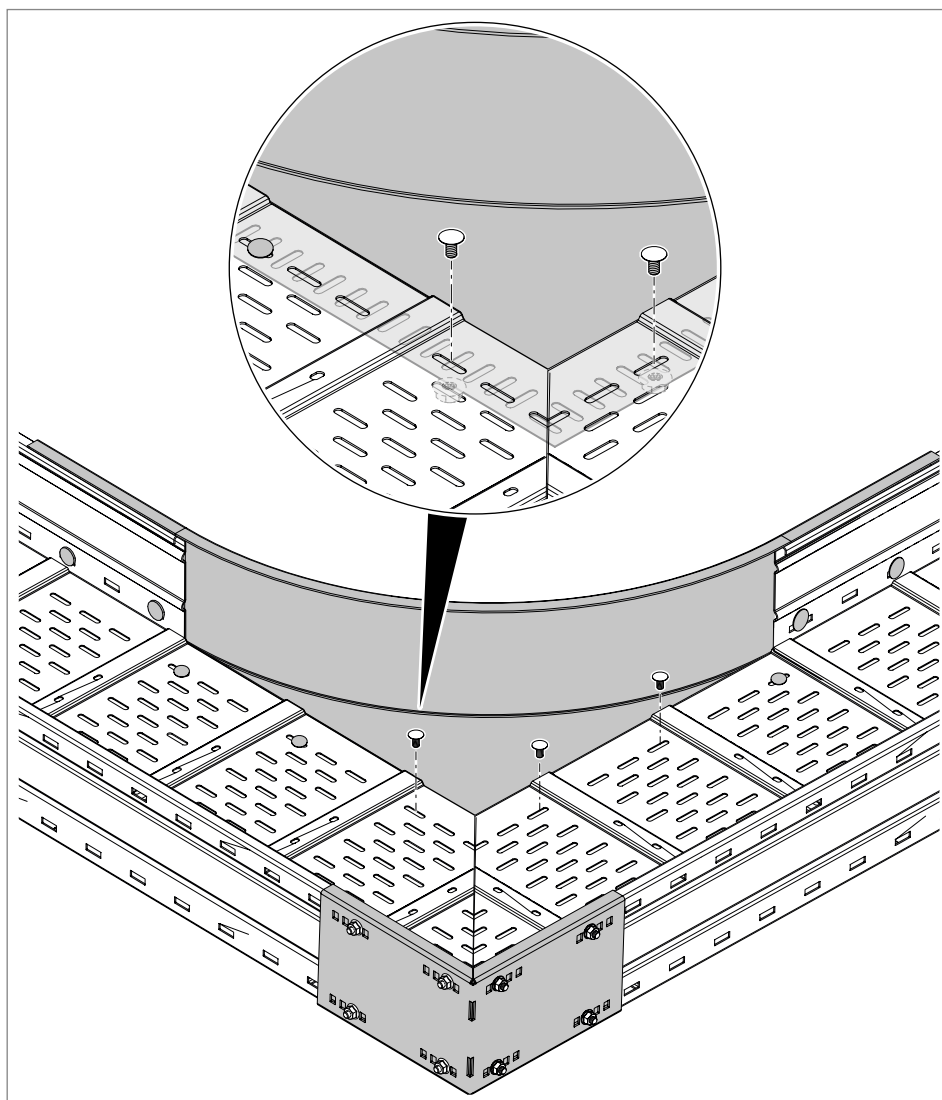
Rys. 42: Przykręcanie listwy stykowej
