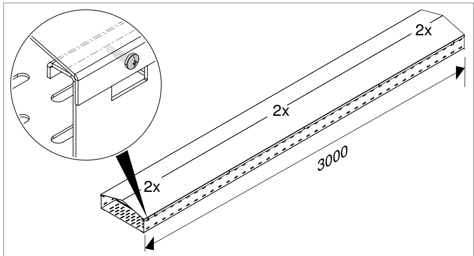
Rys. 44: Pokrywę należy przykręcić w co najmniej 6 miejscach
