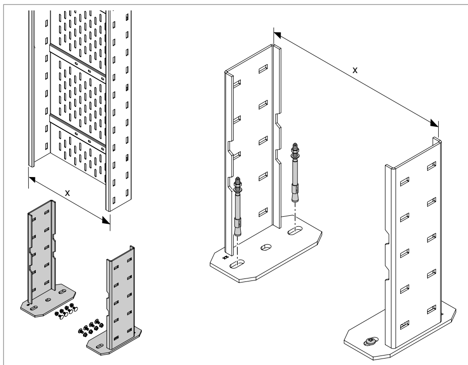
Rys. 28: Podnózek WFP
