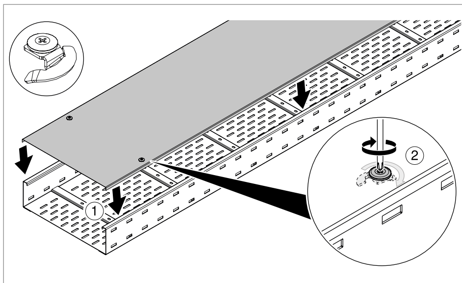
Rys. 45: Zakładanie pokrywy WDRL na szerokorozpięściowe koryto kablowe
