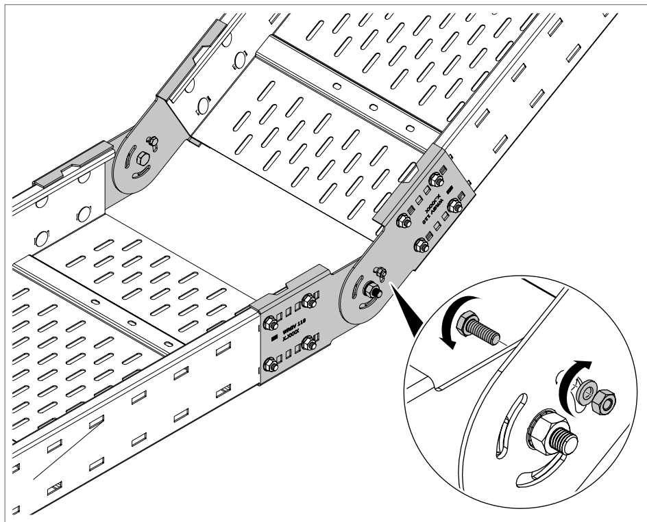
Rys. 24: Montaż koryta wznoszącego
