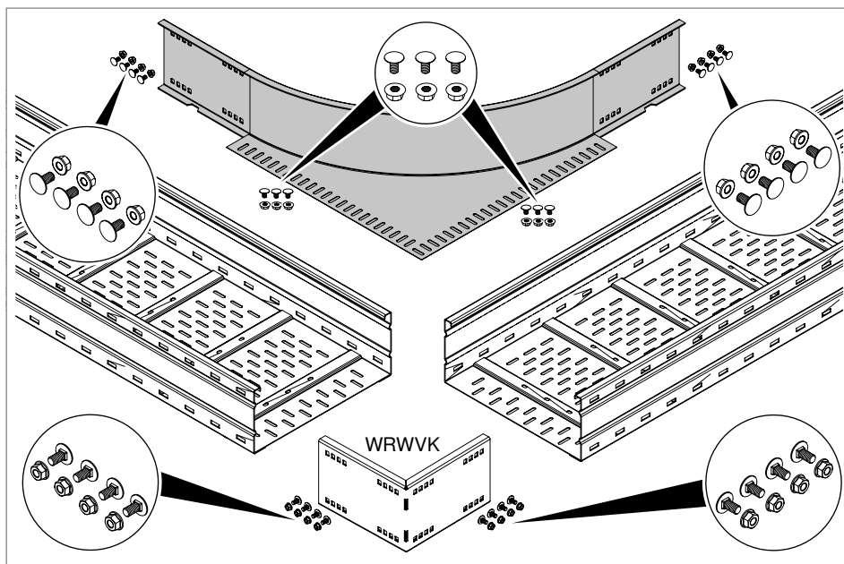
Rys. 39: Komponenty do montażu dołączalnego elementu narożnego WEAS
