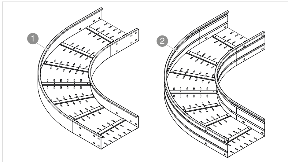
Rys. 4: Łuki 90°
