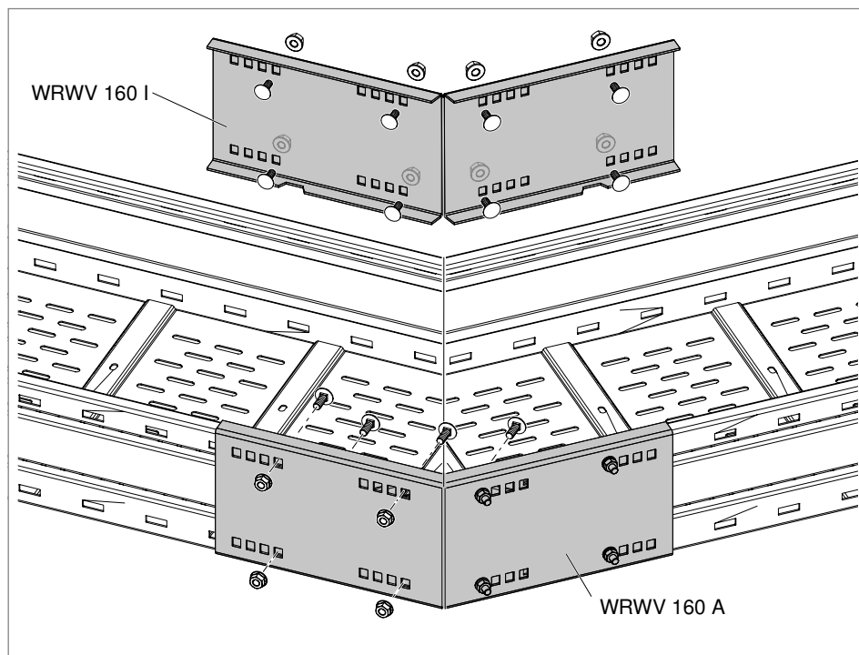
Rys. 15: Przykręcanie łącznika kąowego WRWV do narożnika wewnętrznego i zewnętrznego
