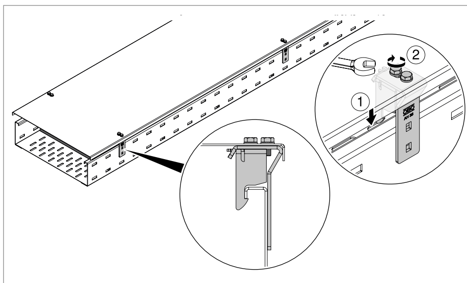
Rys. 49: Montaż pokrywy na korycie
