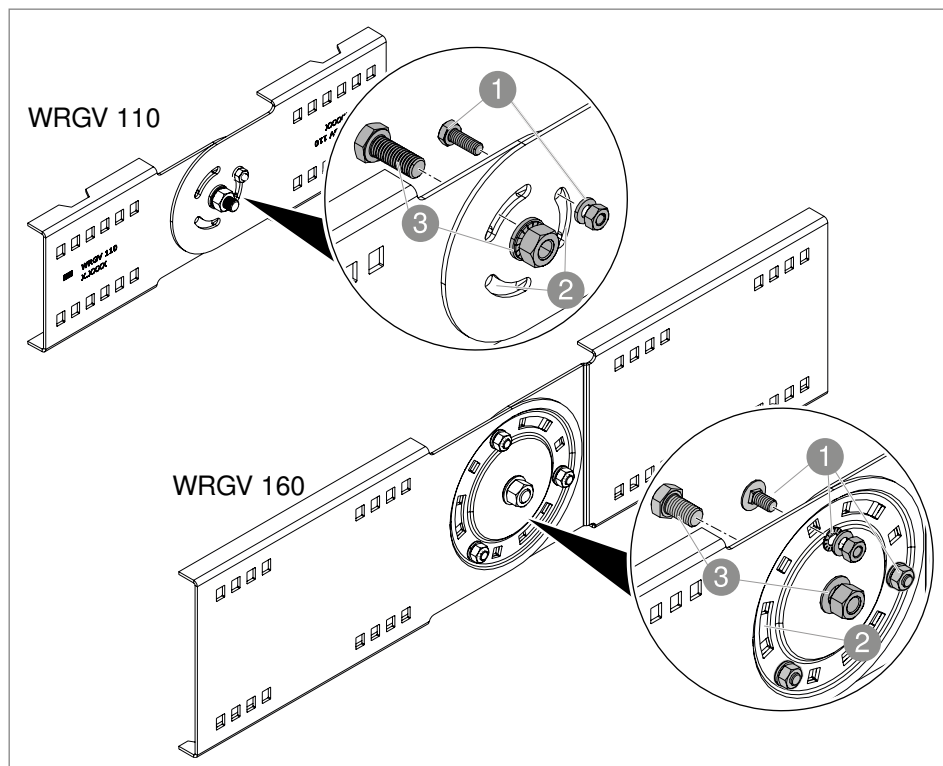
Rys. 21: Przegląd łączników przegubowych WRGV
