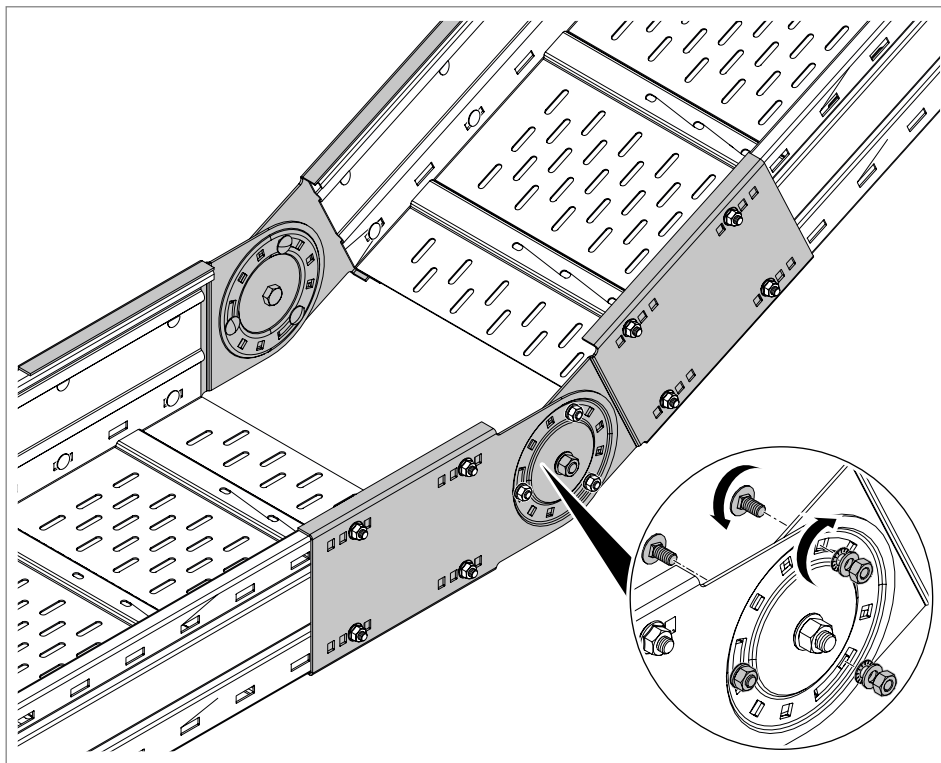
Rys. 27: Montaż koryta wznoszącego
