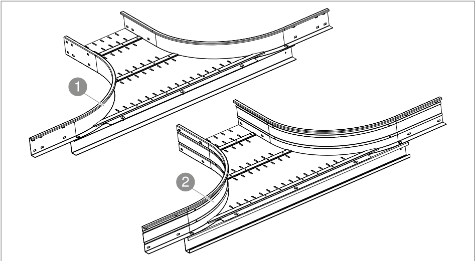
Rys. 6: Trójniki dostawne
