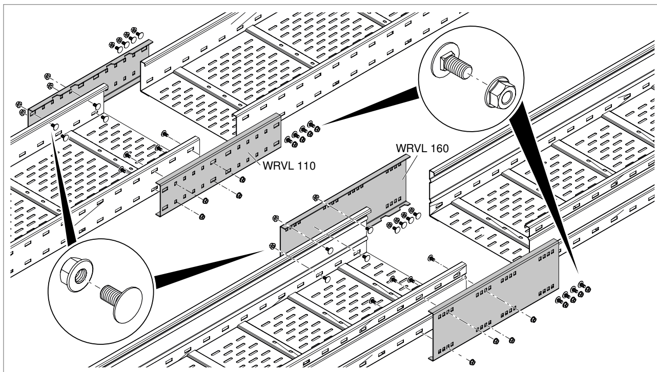
Rys. 10: Zakładanie łącznika wzdłużnego WRVL 110 i 160
