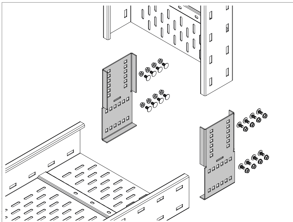
Rys. 19: Łącznik kątowy- pionowy WRWVV
