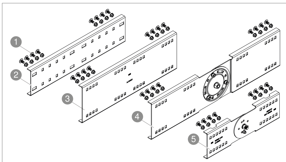
Rys. 2: Łączniki wzdłużne i przegubowe
