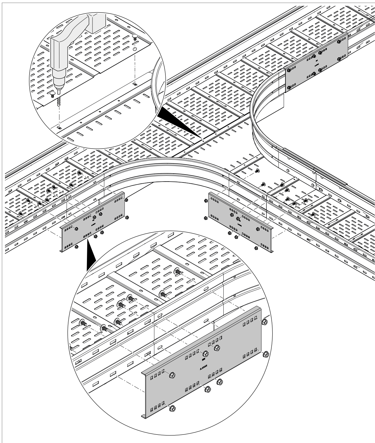
Rys. 37: LDokręcanie łącznika wzdłużnego
