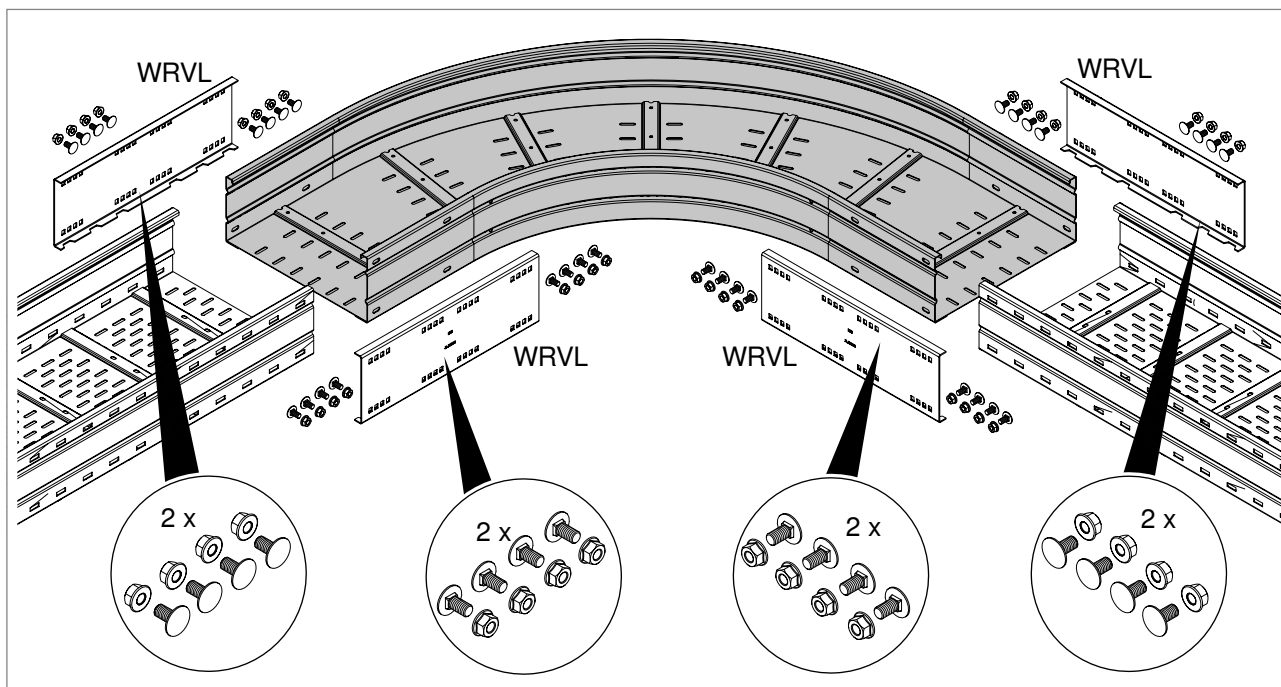
Rys. 32: Elementy do montażu łuku 90°, wysokość boczna 160 mm
