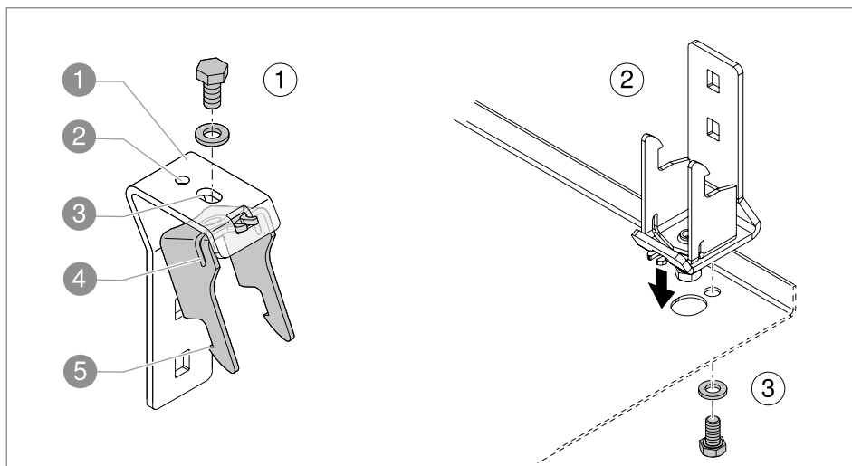
Rys. 47: Montaż elementu dystansowego na pokrywie
