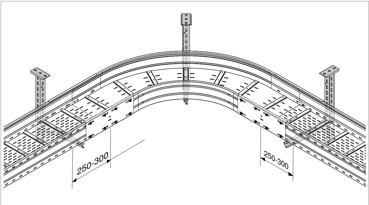
Rys. 31: Przykład: podparcie łuku 90° o szerokości 400 mm
