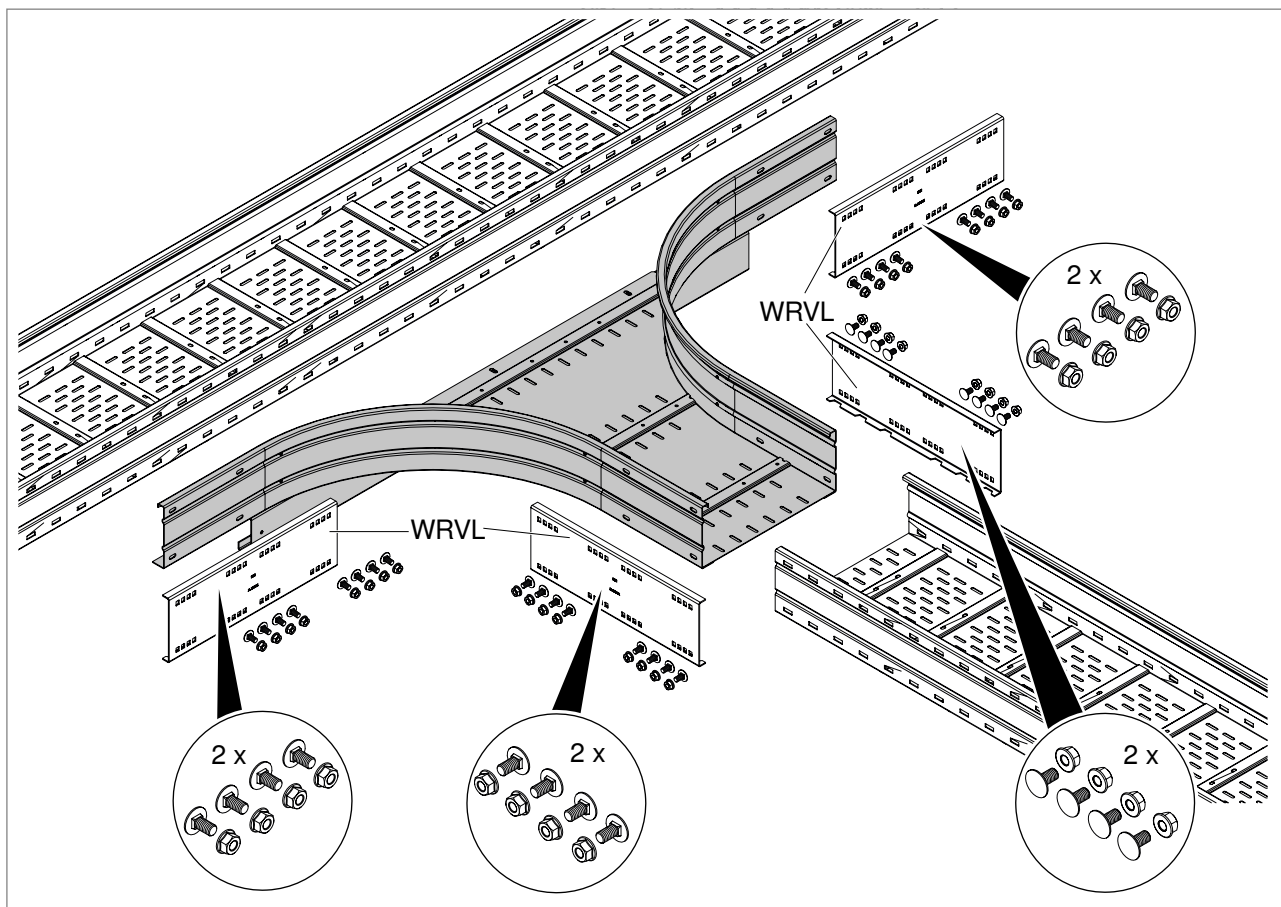
Rys. 35: Komponenty do montażu trójnika dostawnego
