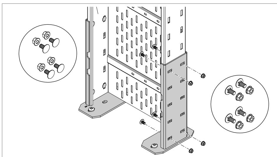
Rys. 29: Przykręć korytko kablowe do podnózek
