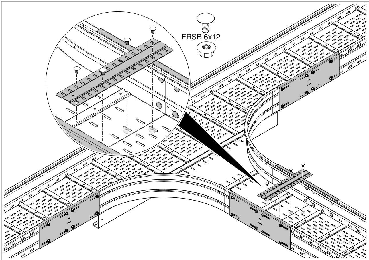
Rys. 38: Przykręcanie listwy stykowej
