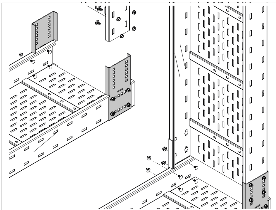
Rys. 20: Przykręcanie łącznika kąтового WRWVV
