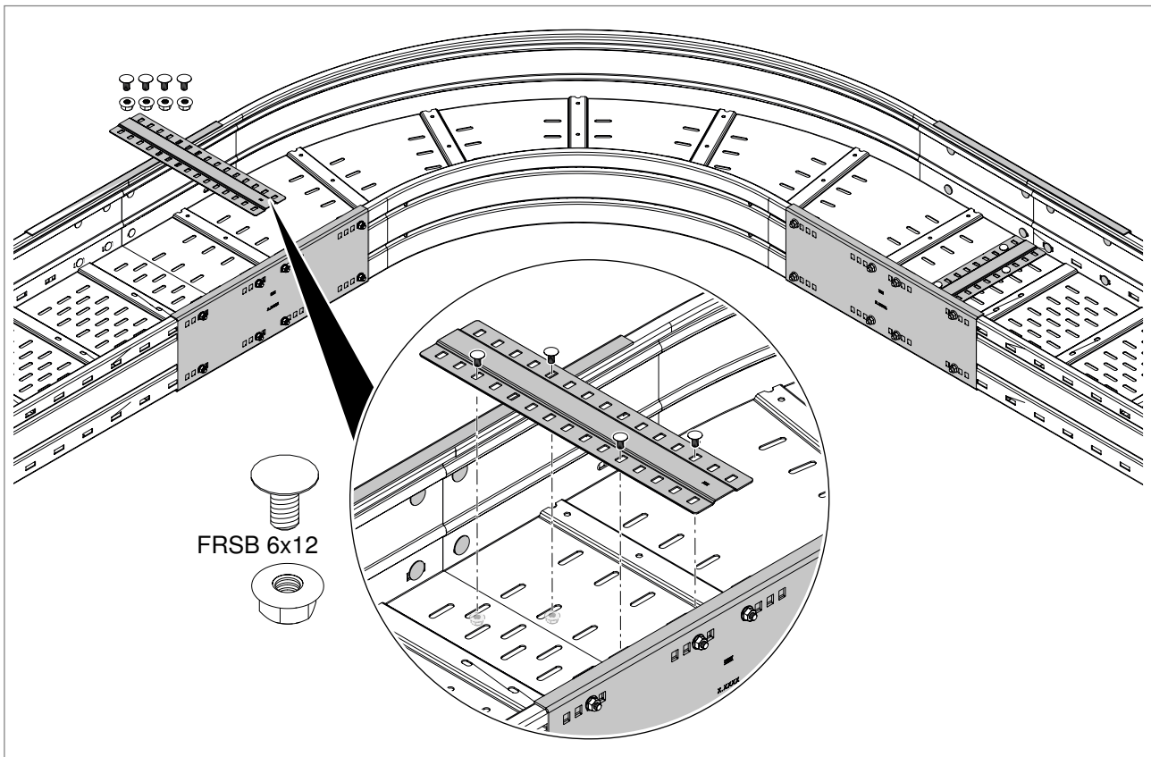
Rys. 34: Przykręcanie listwy stykowej
