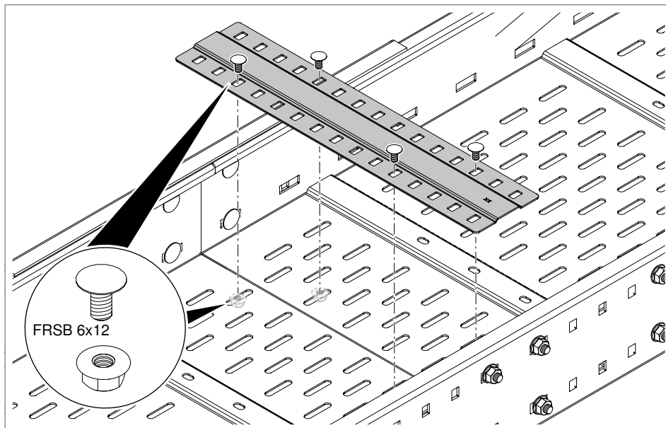
Rys. 12: Montaż listwy stykowej
