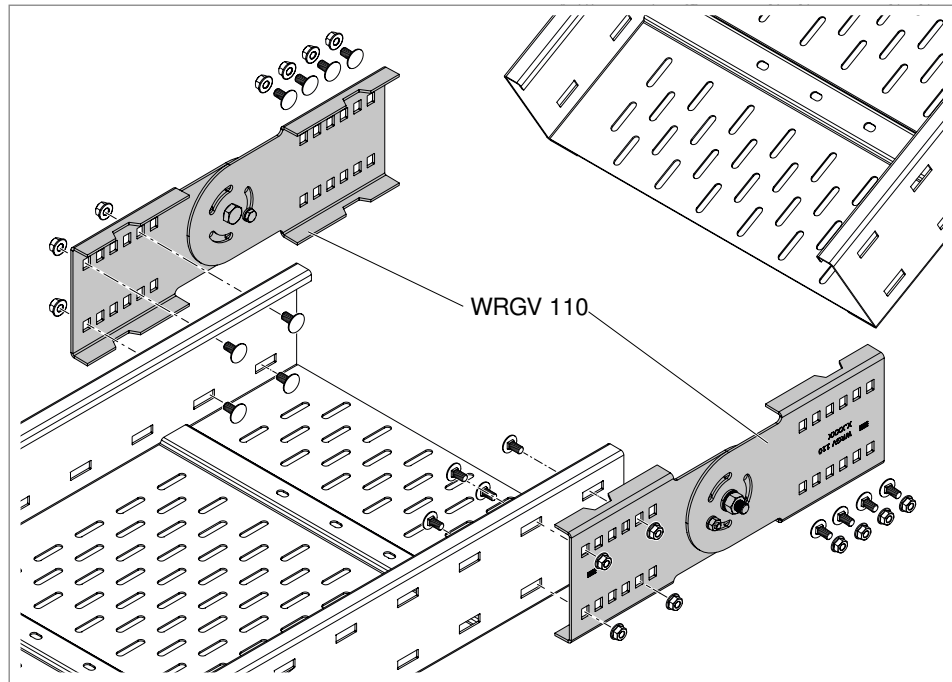
Rys. 22: Zakładanie łącznika przegubowego
