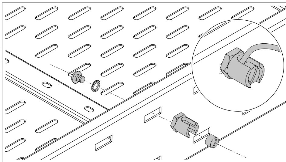
Rys. 50: Montaż zacisku uziemiającego
