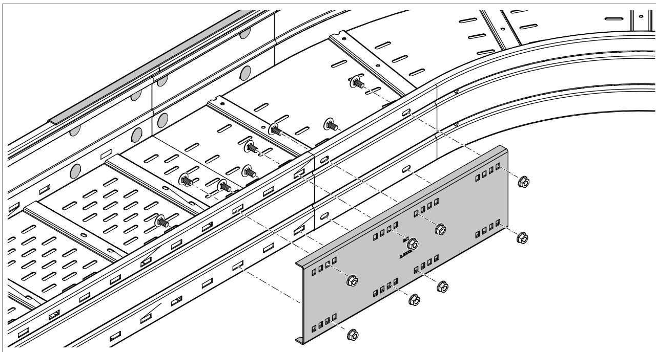
Rys. 33: Przykręcanie łączników
