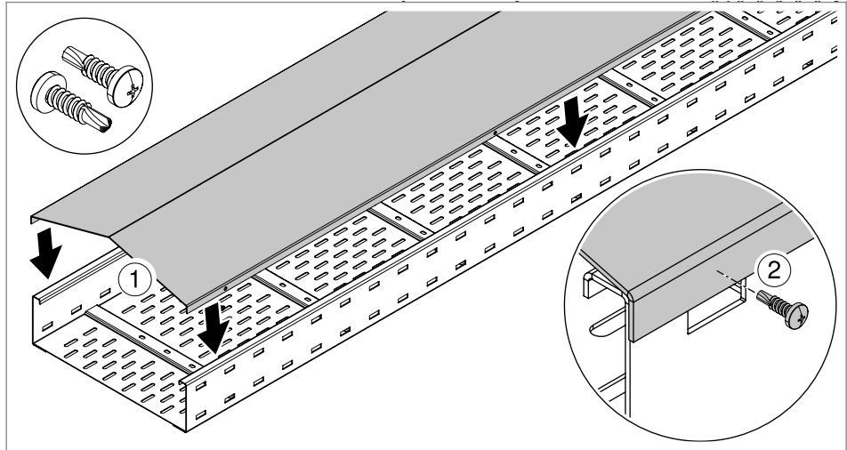
Rys. 43: Zakładanie pokrywy WDRLU DF na szerokorozpiętościowe koryto kablowe
