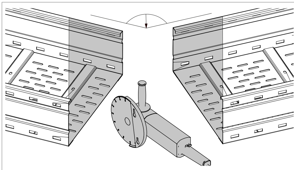
Rys. 14: Przycinanie koryt do ustawienia kątowego
