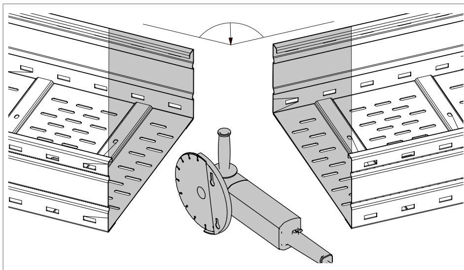
Rys. 16: Przycinanie koryt do ustawienia kąтового
