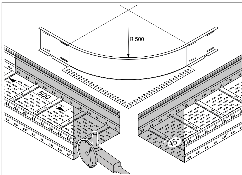
Rys. 40: Nacinanie szerokorozpięściowego koryta kablowego do montażu dołączalnego elementu narożnego
