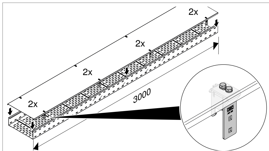
Rys. 48: Zamontowany element dystansowy na pokrywie DRL FAM
