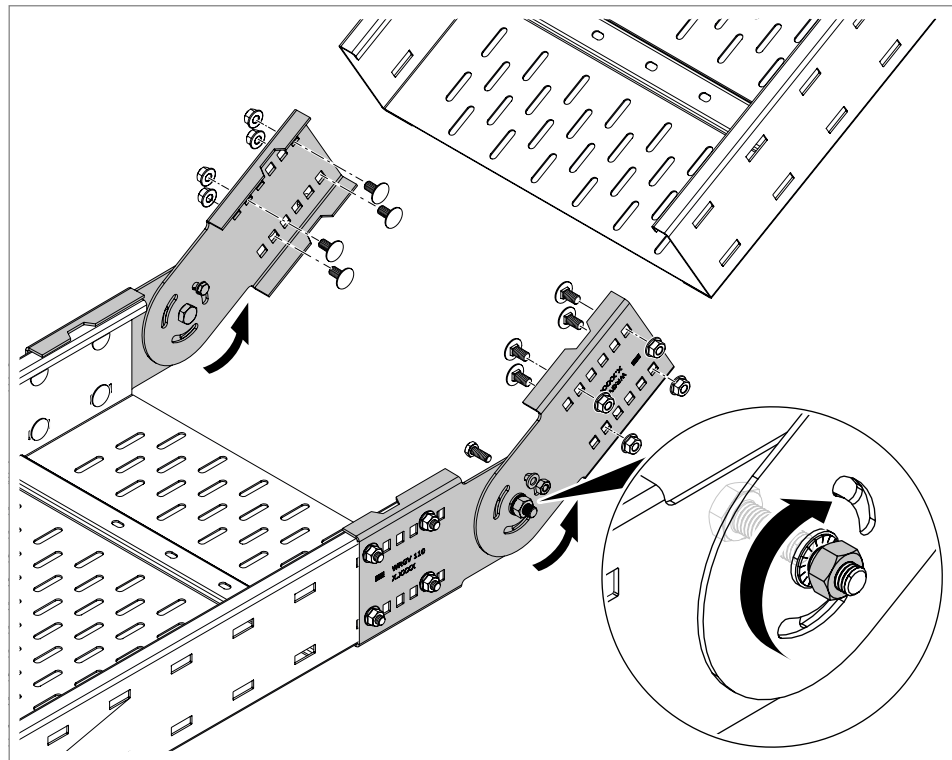
Rys. 23: Ustawianie kąta
